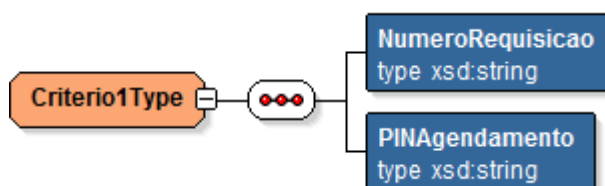
Fig. 29- Estrutura Critério1Type.
