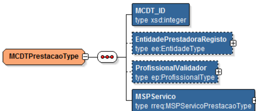
Fig. 10 - Estrutura MCDTPrestacaoType.
