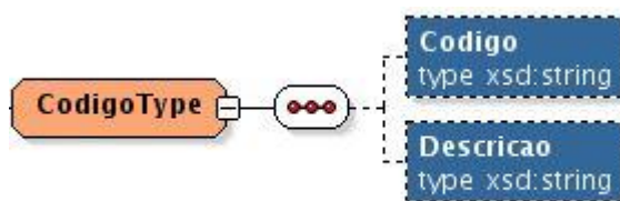
Fig. 22- Estrutura CodigoType.
