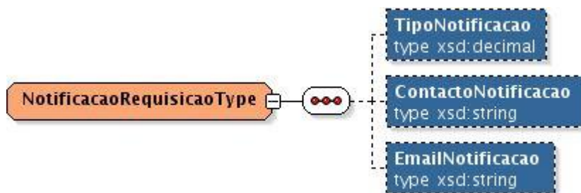
Fig. 40- Estrutura NotificacaoRequisicaoType
