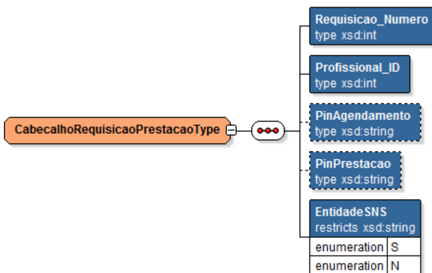
Fig. 17 - Estrutura CabecalhoRequisicaoPrestacaoType.
