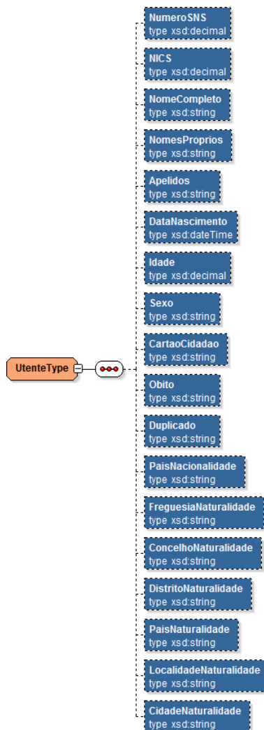
Fig. 12- Estrutura UtenteType.
